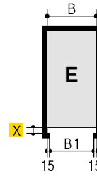
Reihengarage mit Einzeltoren
